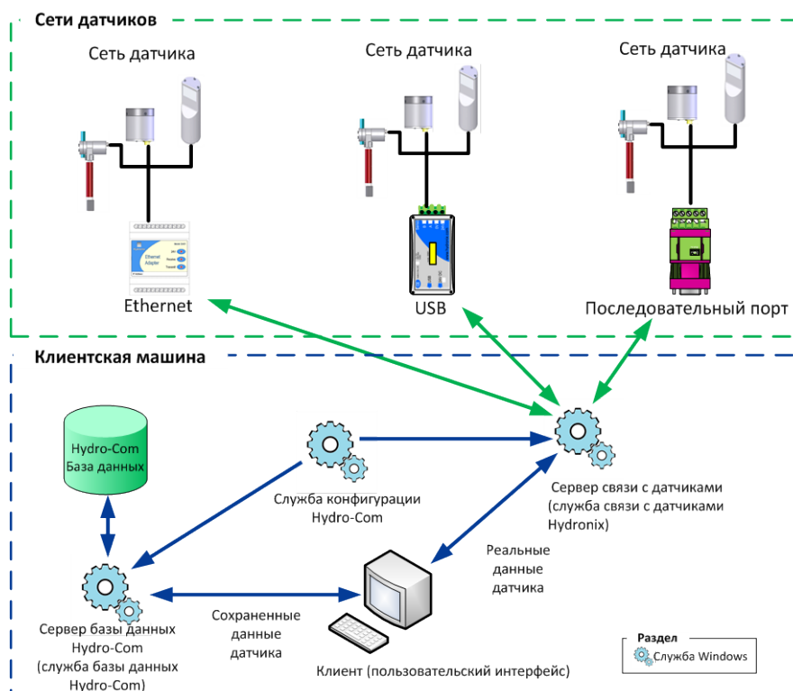
Рис. 1: Обзор системы Hydro-Com
