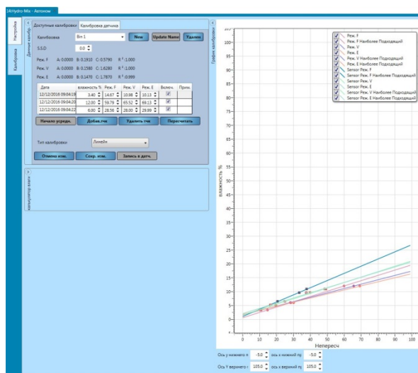
Рис. 21: График калибровки
