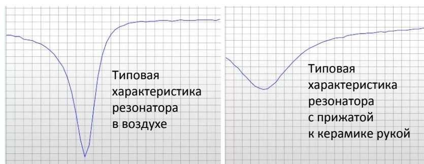
Рис. 42: Типовая характеристика резонатора
