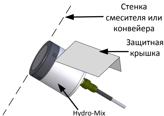
Рисунок 17: Датчик Hydro-Mix с защитной крышкой
