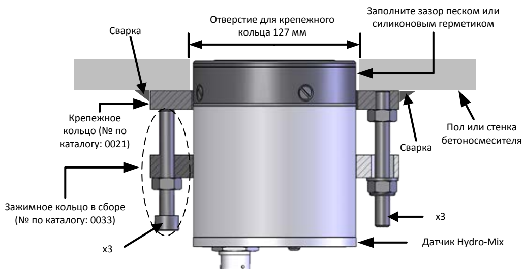
Рисунок 11: Монтаж датчика
