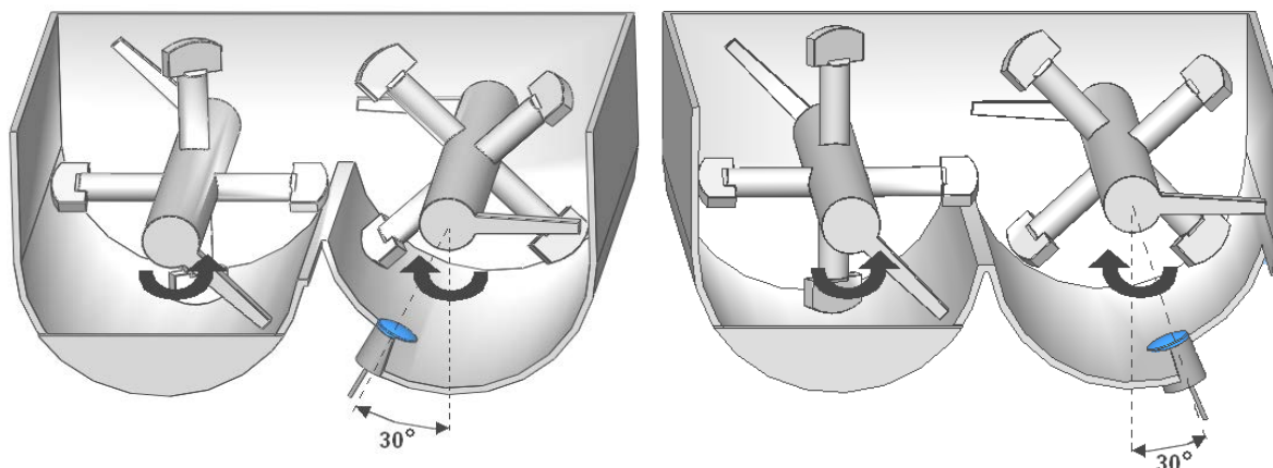
Рисунок 7: Монтаж в двухвальном бетоносмесителе
