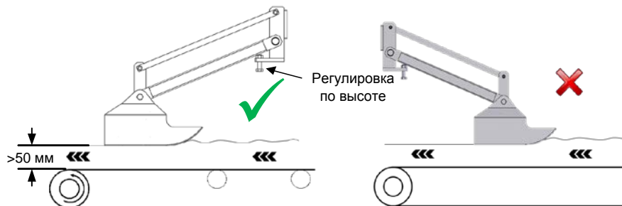
Рисунок 10: Монтаж датчика Hydro-Skid на ленточном конвейере
