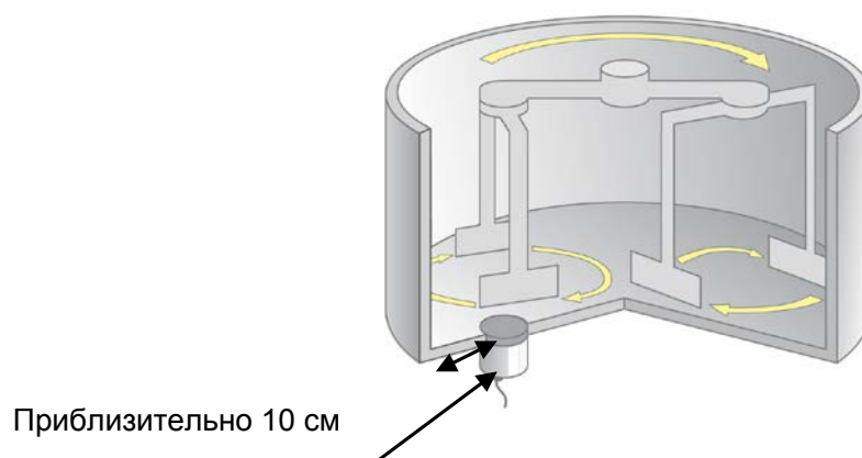
Рисунок 5: Монтаж в планетарном бетоносмесителе
