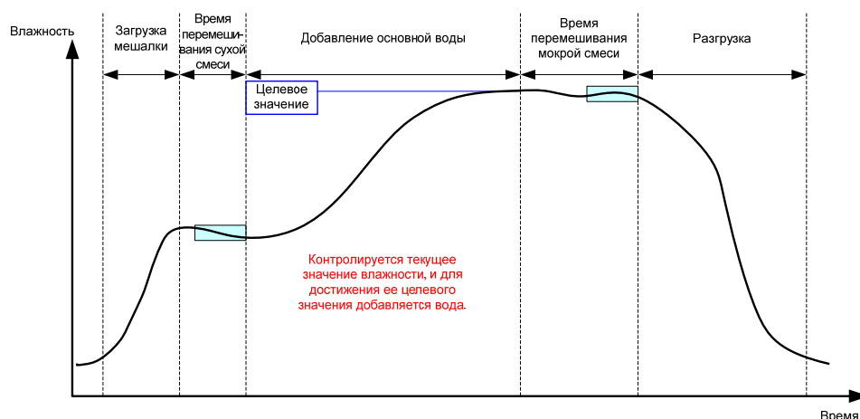
Рис. 22: Изменение влажности в режиме Автоматический
