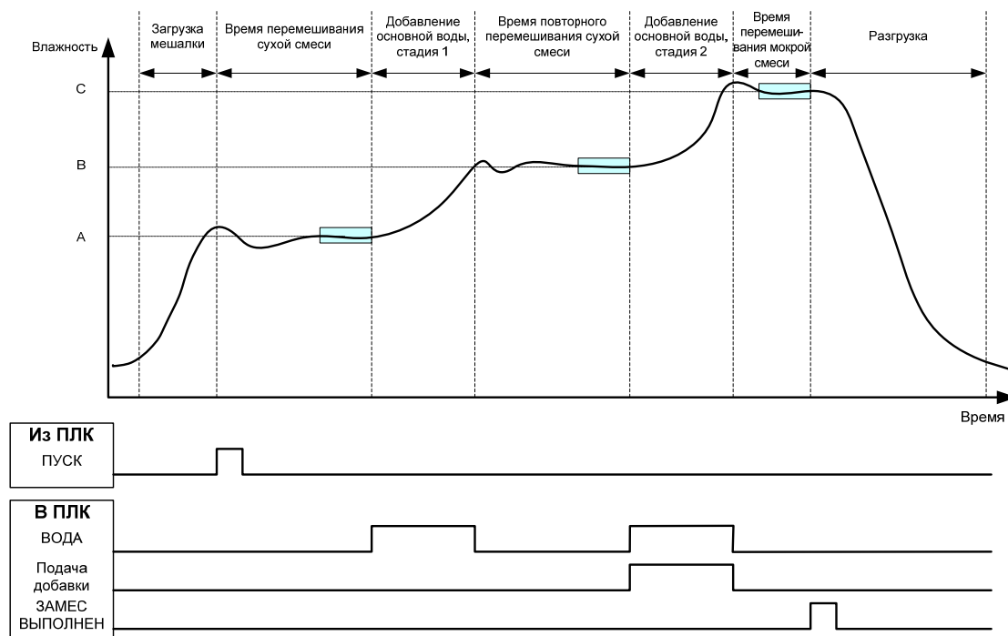
Рис. 26: Цикл 2-ступенчатого режима Заданный
