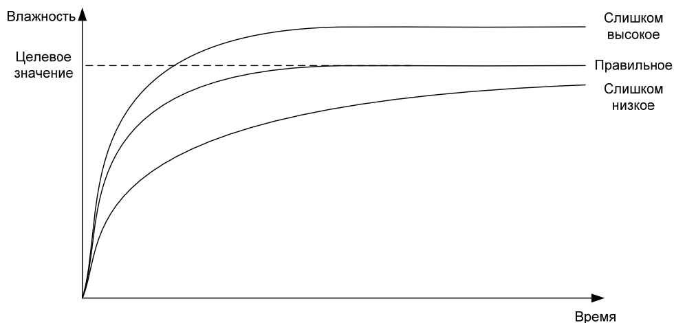
Рис. 23: Эффект изменения коэффициента пропорциональности
