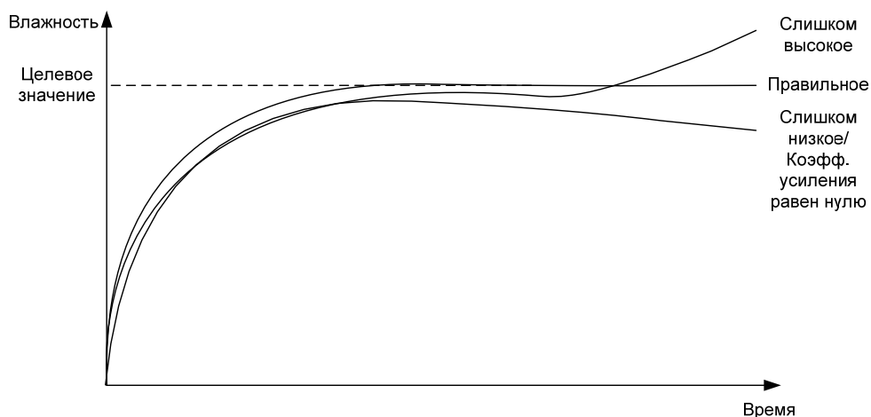
Рис. 24: Эффект изменения интегрального коэффициента регулятора
