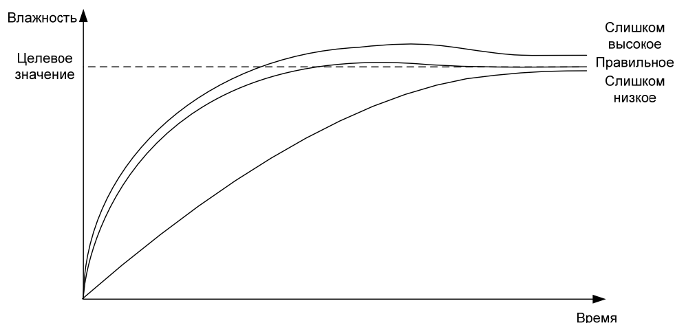
Рис. 25: Эффект изменения коэффициента пропорциональности
