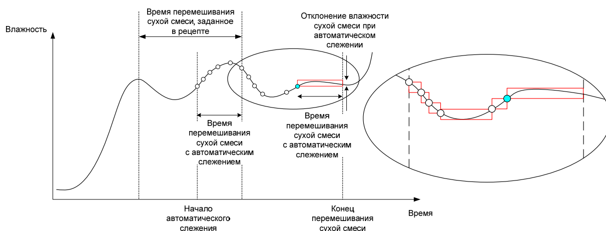
Рис. 28: График замеса, отображающий функцию автоматического слежения
