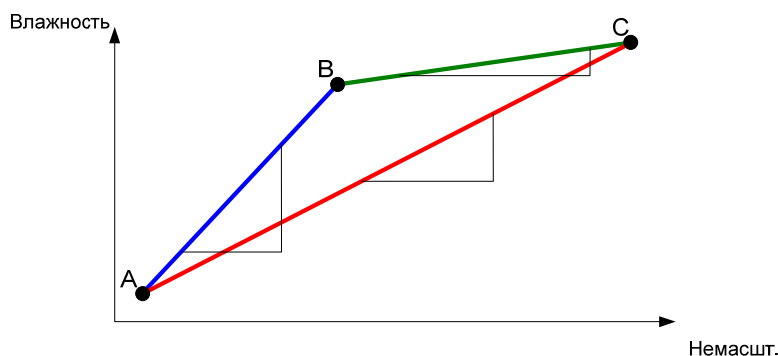
Рис. 27: Линии калибровки для 2-ступенчатого цикла в режиме Заданный
